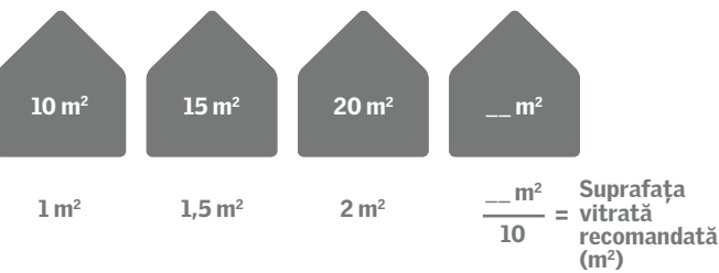
Regula de bază în iluminatul natural
